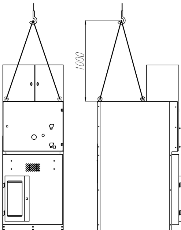
Рис. 5.1 Схема строповки
