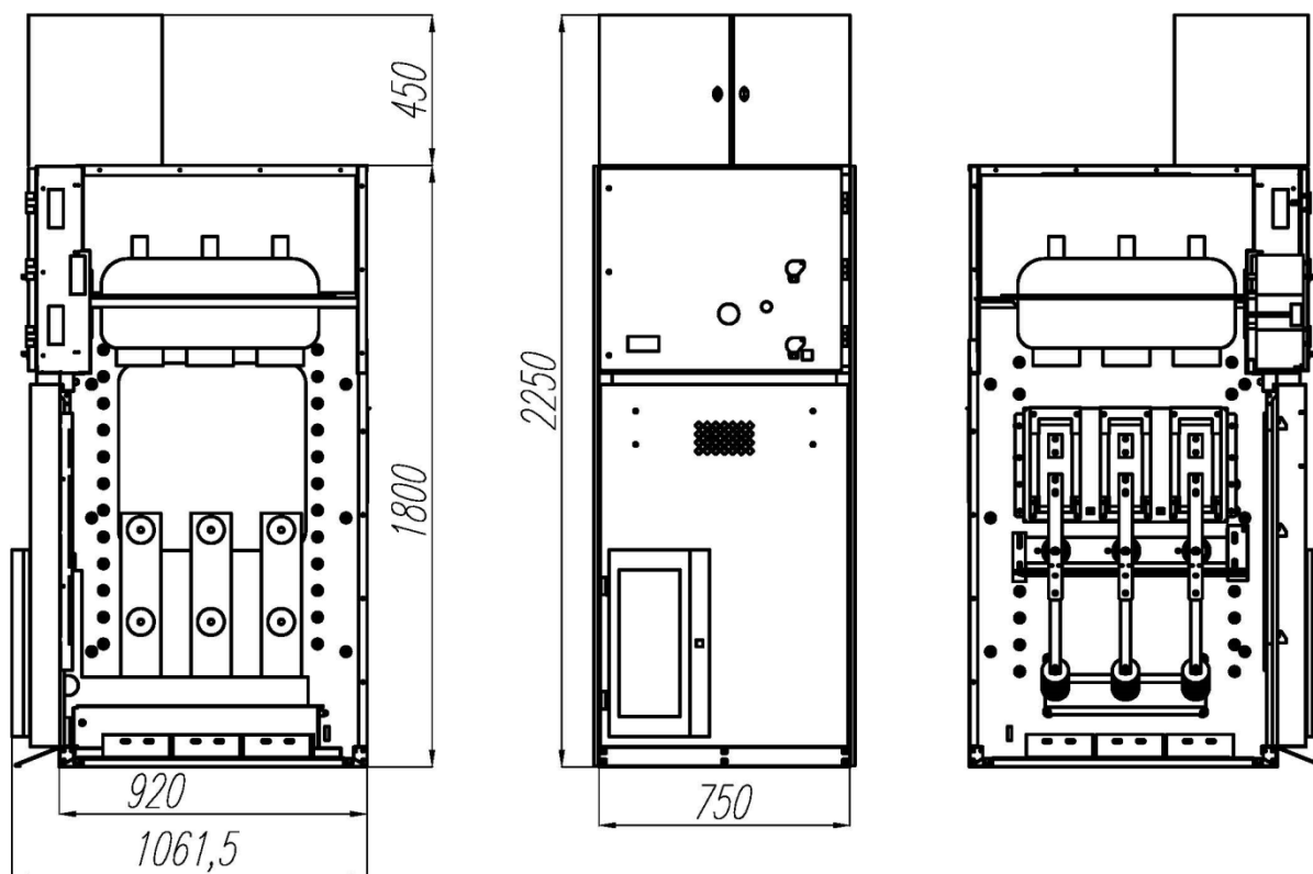
Рис. 2.7 Габаритные размеры ячейки КСО СЕРИИ «ИРИС» (функцияV)
