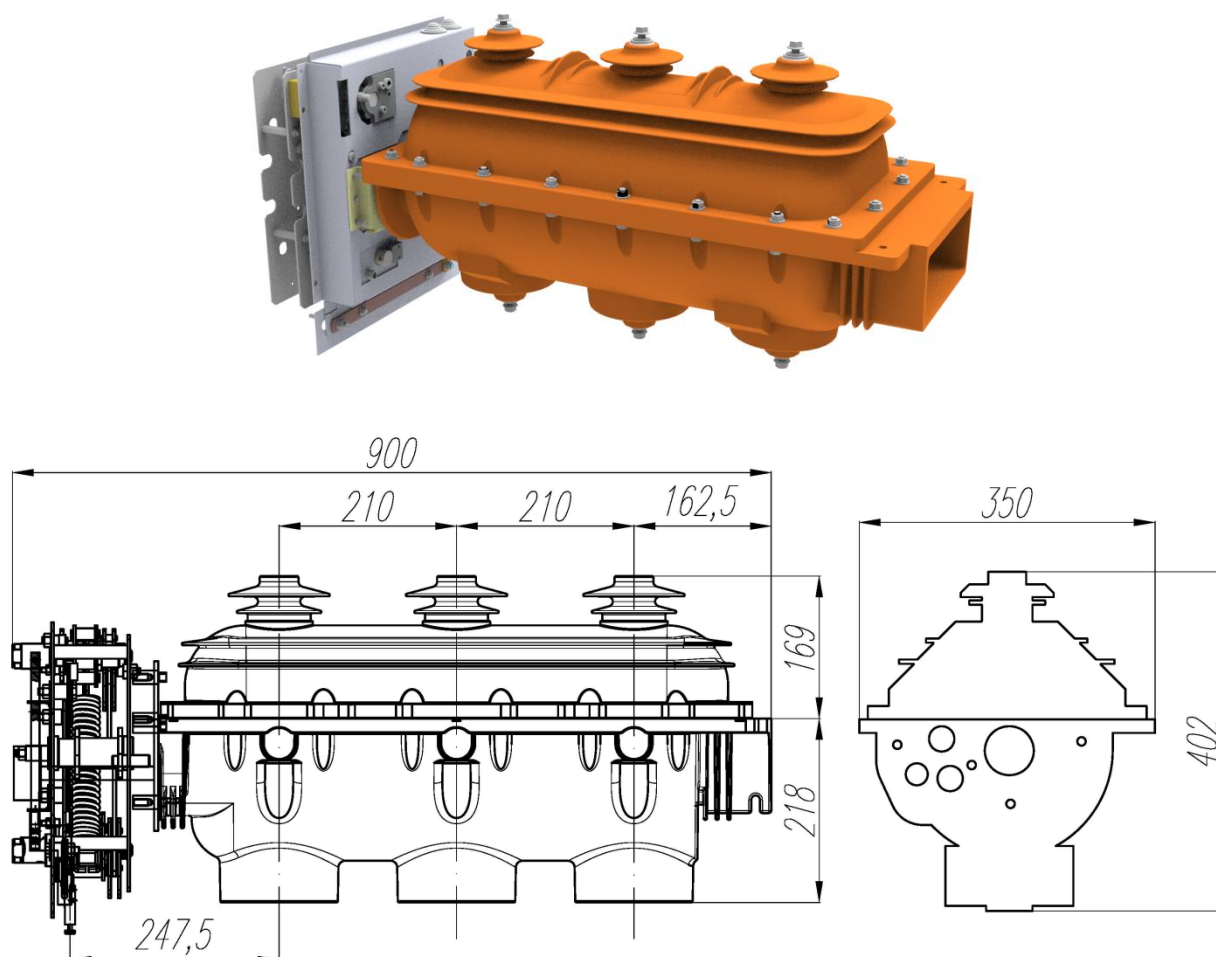
Рис. 2.2 Элегазовый ВН
