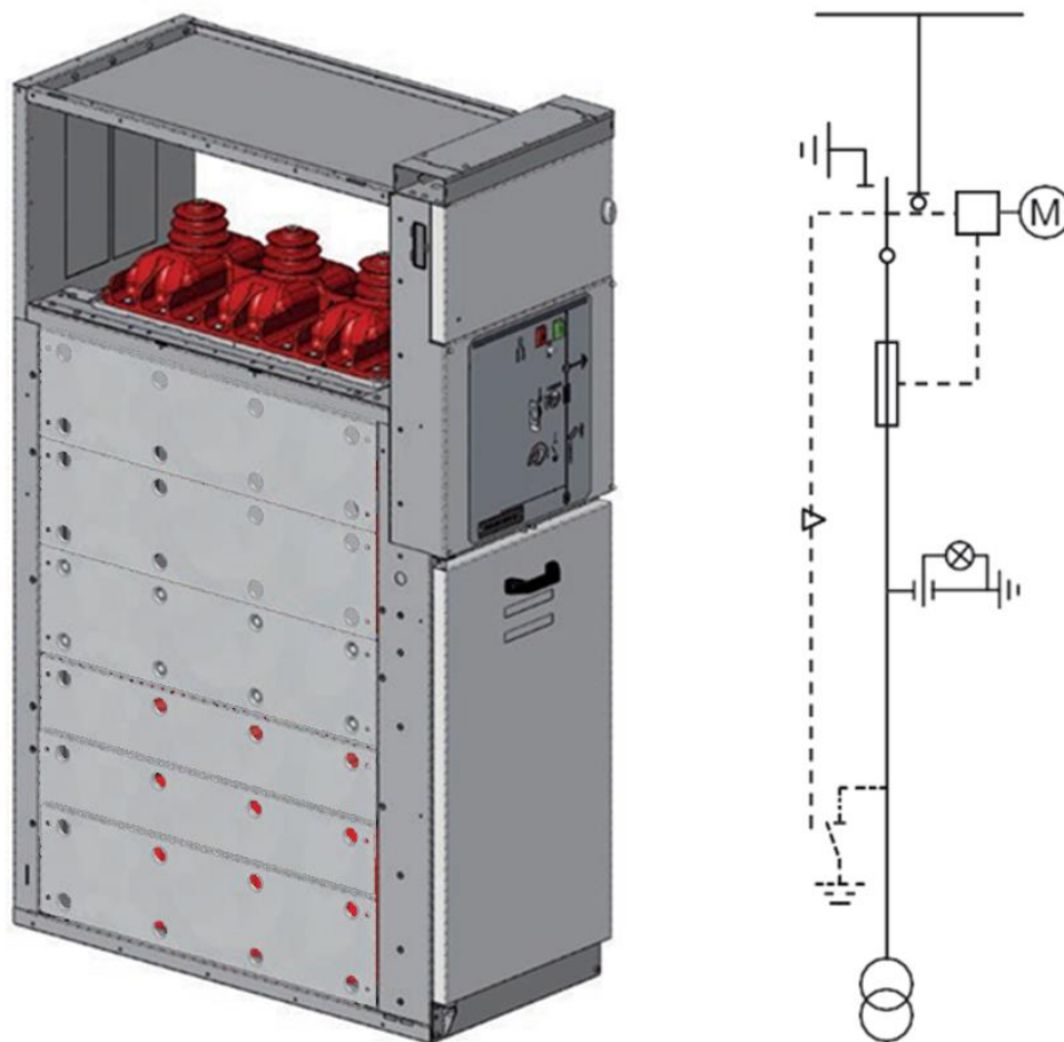
Рис. 2.6 Внешний вид и однолинейная схема функции Cvt
