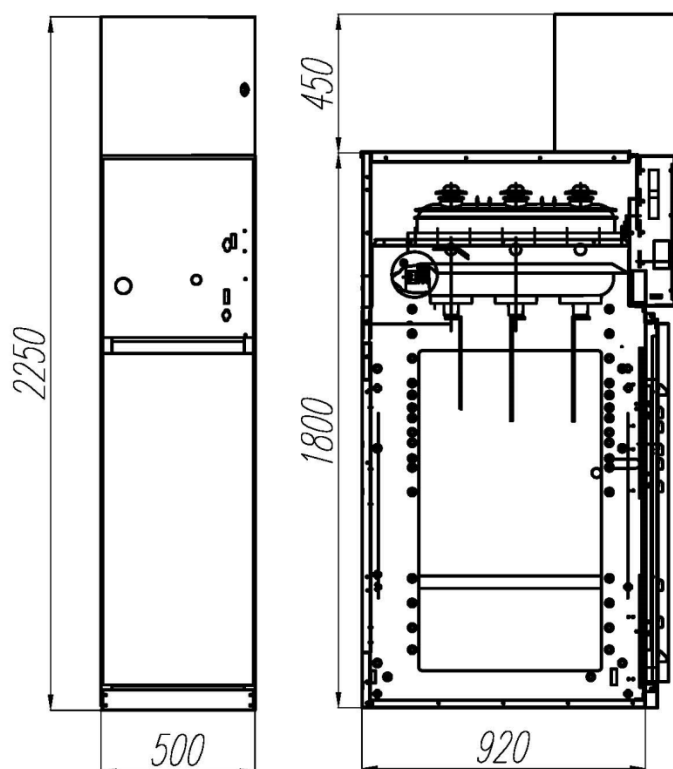
Рис. 2.8 Габаритные размеры ячейки КСО СЕРИИ «ИРИС» (функцияС, Cvt)
