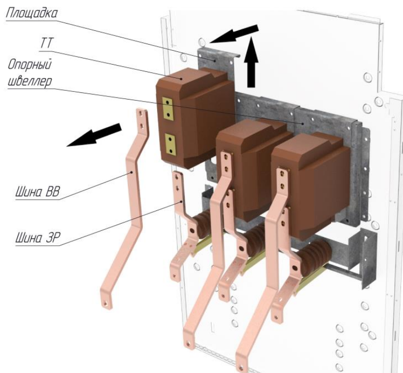
Рис. 7.1 Замена ТТ
