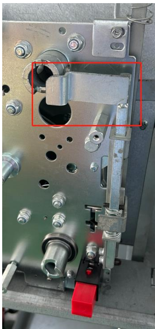
Рис. 6.5 Блокирование включения при открытой крышке кабельного отсека
