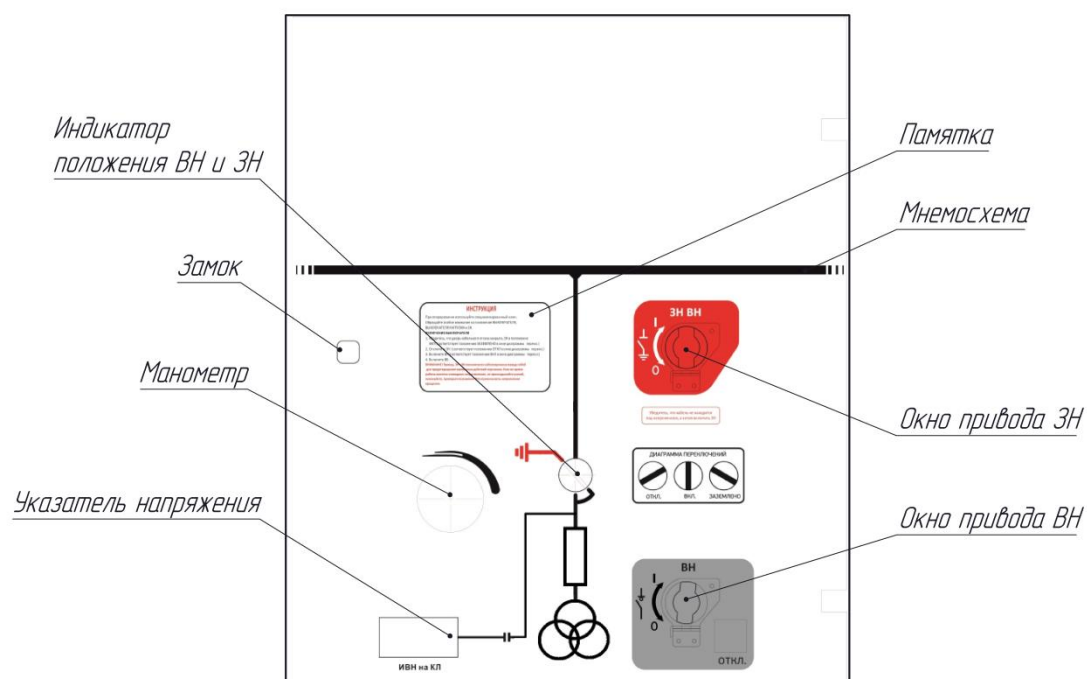
Рис. 6.3 Лицевая панель ВН функции Cvt
