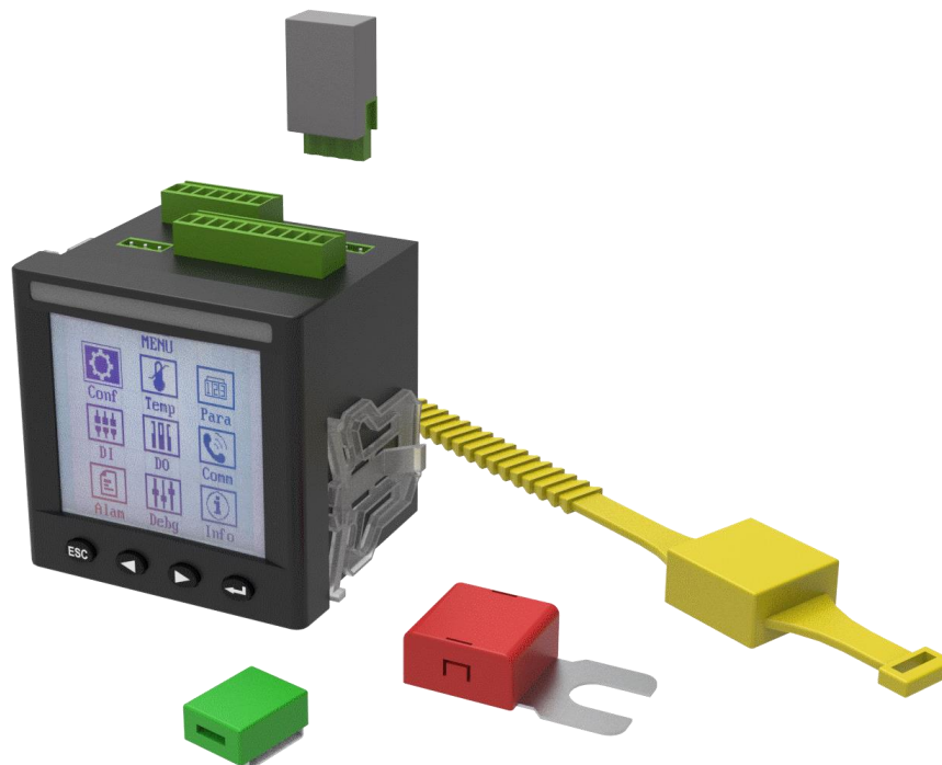
Рис. 8.7 БСКТ
