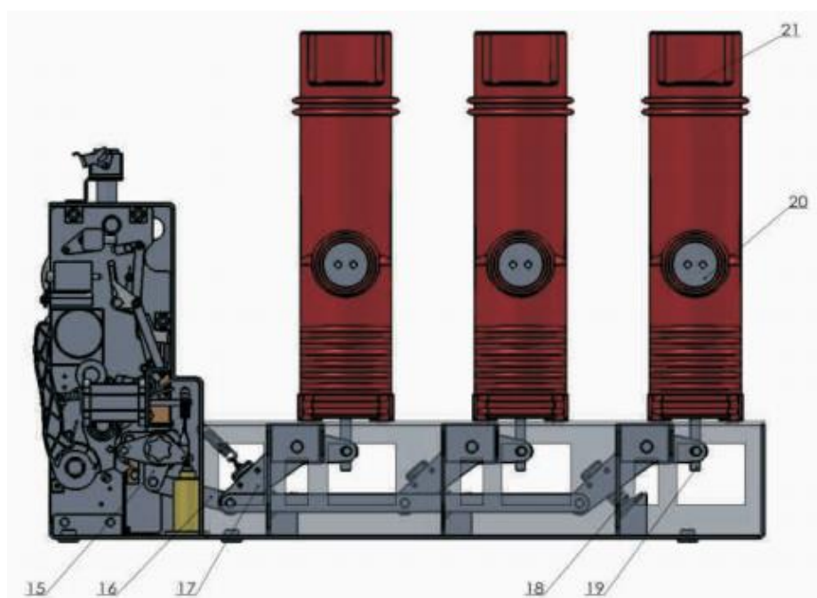
Рис. 2.4. Привод выключателя
