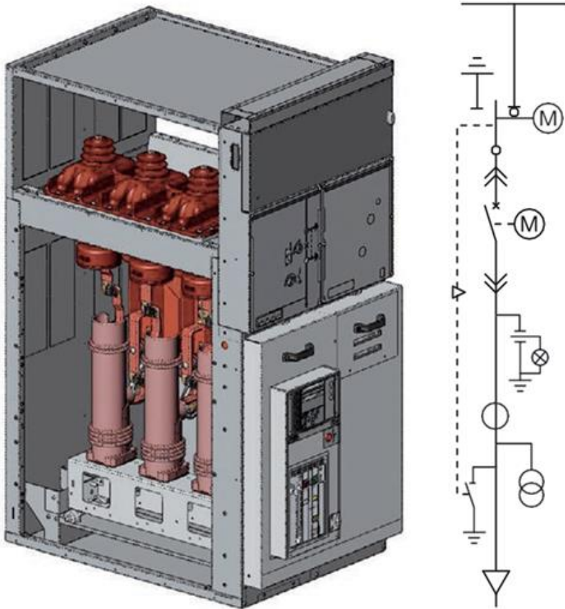
Рис. 2.5 Внешний вид и однолинейная схема функции V
