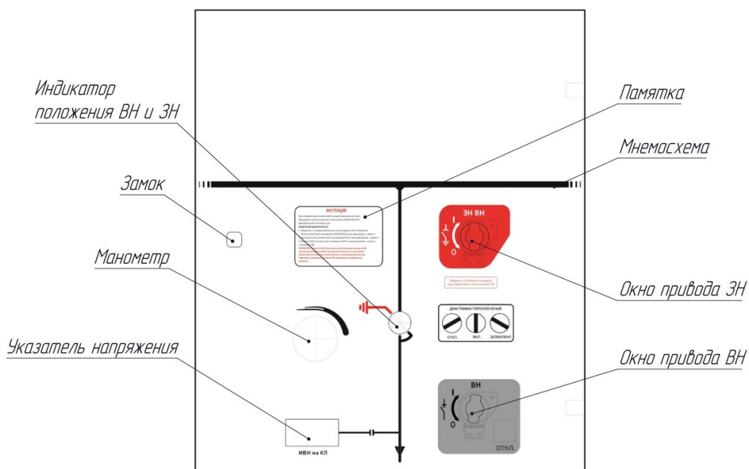
Рис. 6.2 Лицевая панель ВН функции С
