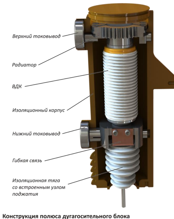
Рис. 2.5 Конструкция полюса дугогасительного блока
