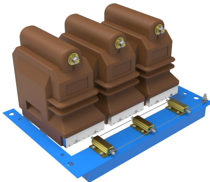
Рис. 8.5 Трансформатор напряжения типа 3хЗНОЛП-НТЗ-10
