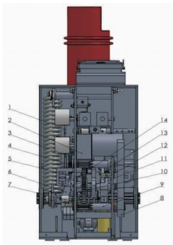
Рис. 2.3 Привод выключателя
