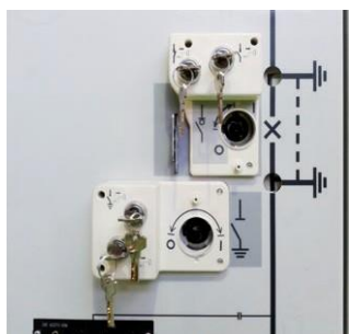
Рис. 6.6 Замки типа Ronis
