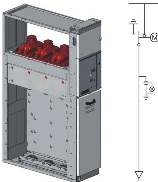
Рис. 2.4 Внешний вид и однолинейная схема функции С
