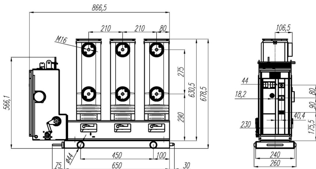
Рис. 2.3 Габаритные размеры вакуумного выключателя
