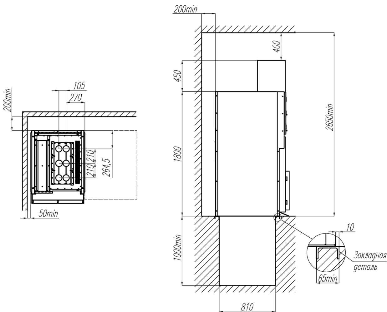
Рис. 5.2 Схема установки
